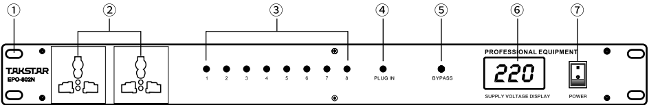
① 安装孔 ② 直通电源输出插座 ③ 电源输出指示灯 ④ 电源指示灯 ⑤ 直通键开关(通断所有通道的输出) ⑥ 输出电压 ⑦ 电源开关
